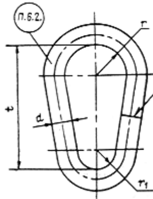
Рис. П.1.10. Звено типа О
